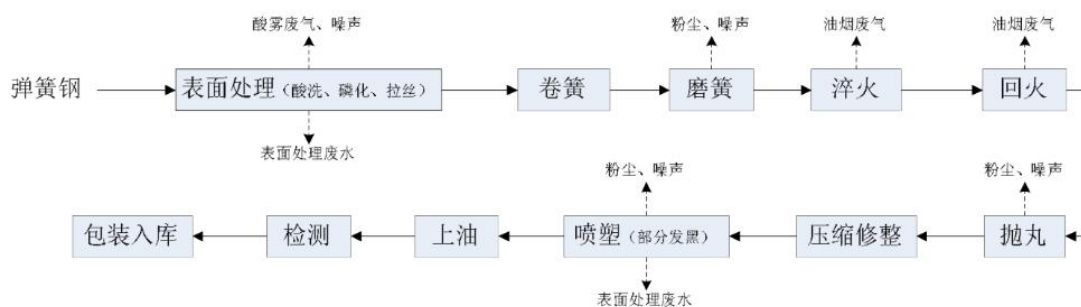
图 4.5-24 弹簧生产工艺流程图
