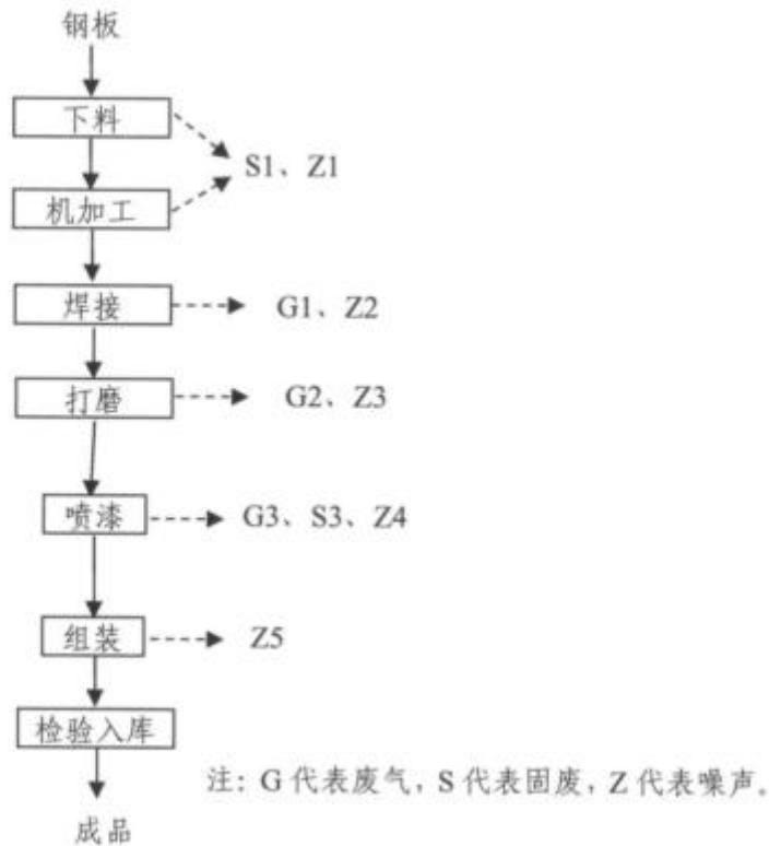
图 4.4-4 升降机械工艺流程
