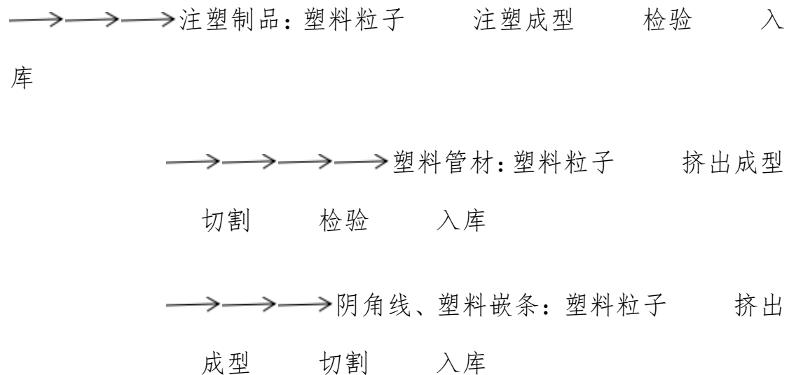
图 4.4-3 工艺流程
