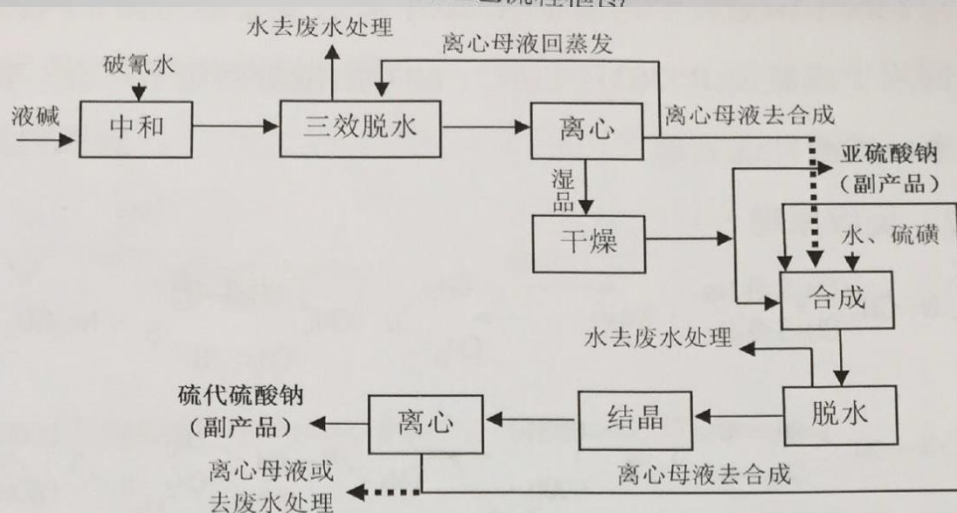
图 1-2 续 杀螟丹原药产品工艺流程框图
