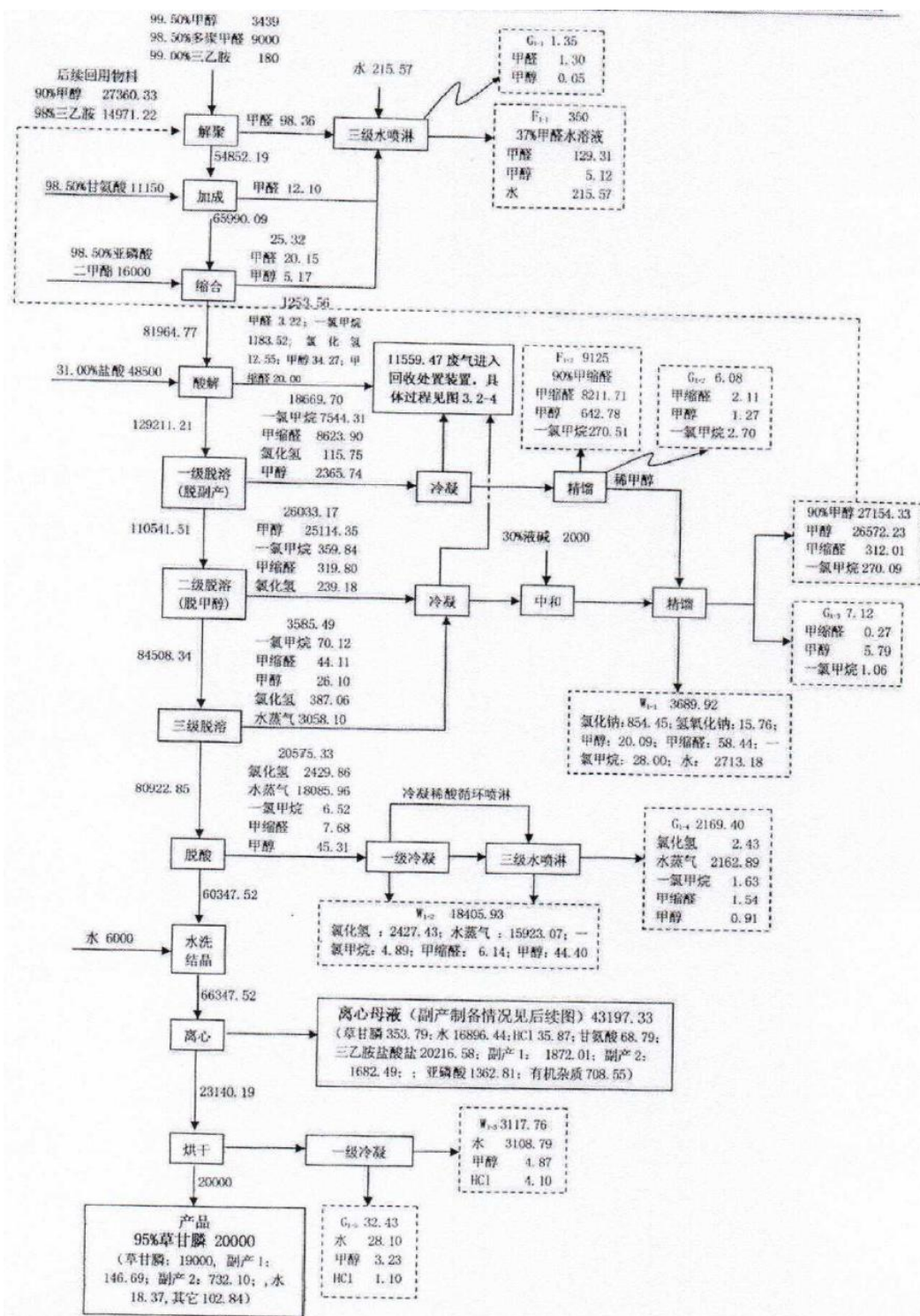
图 3.2-1 年产 20000 吨草甘膦项目物料平衡图 单位: t/a
