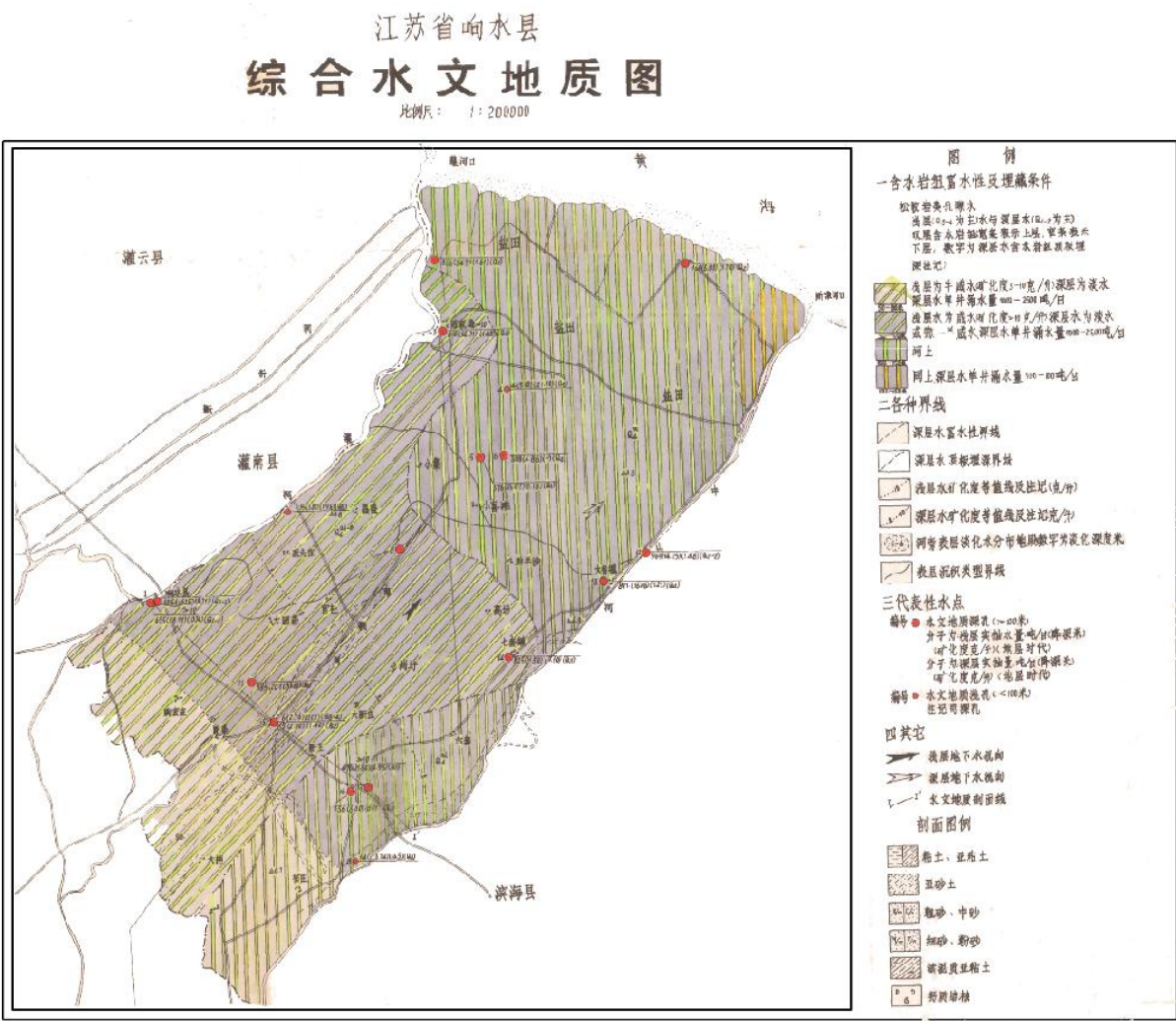
图 3.1.6-3 响水县综合水文地质图
