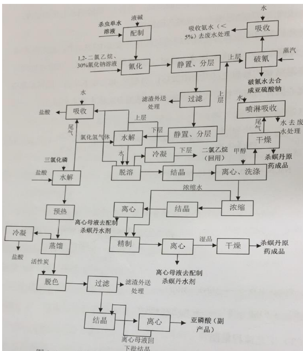
图 1-2 杀螟丹原药产品工艺流程框图
