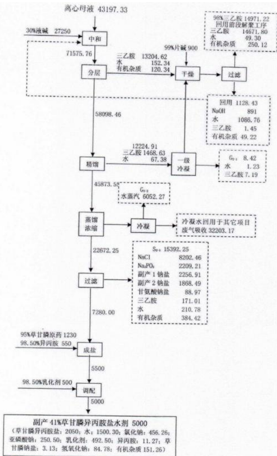
图 3.2-2 年产 5000 吨 41%草甘膦异丙胺盐水剂项目物料平衡图 单位: t/a
