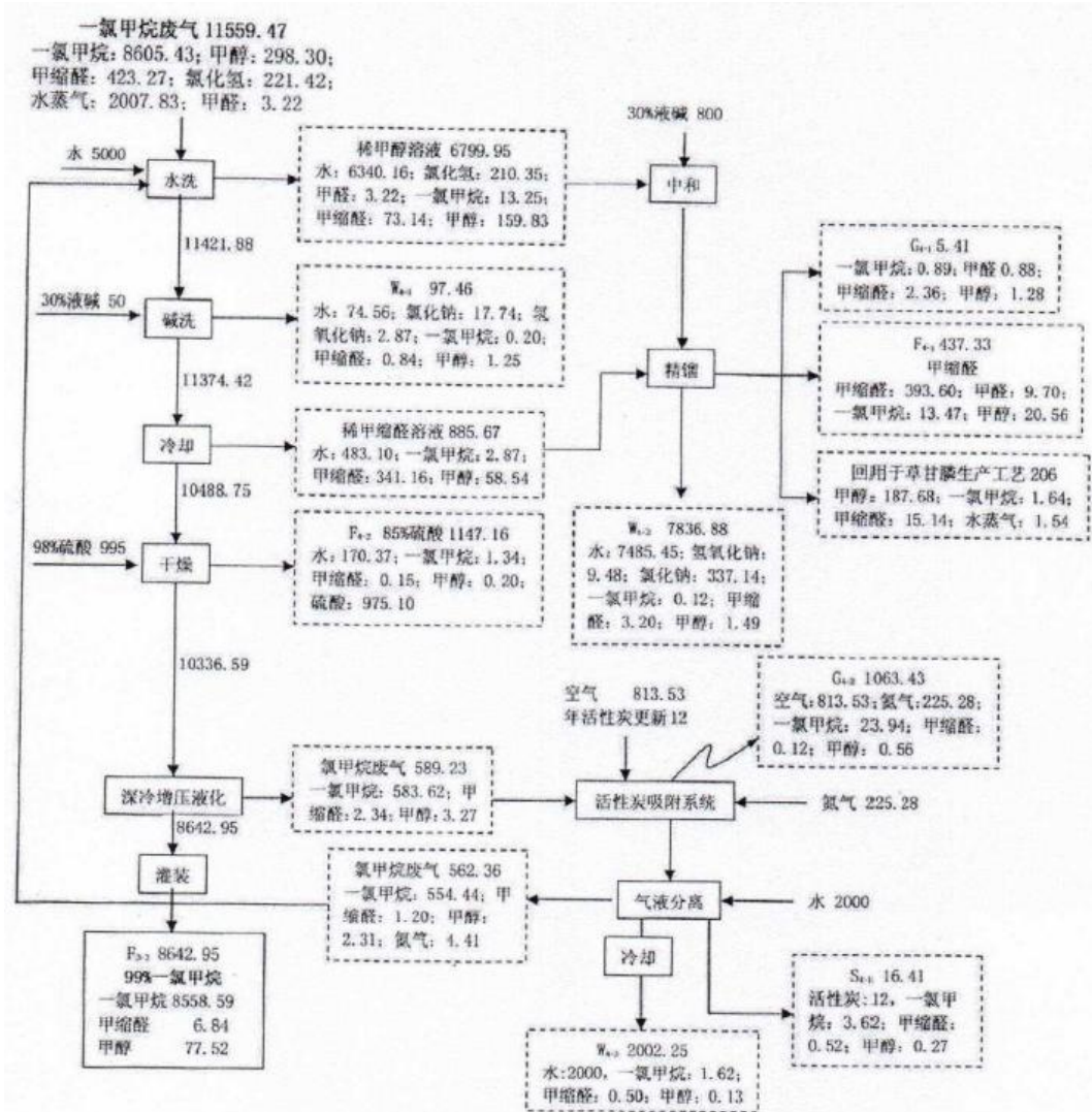
图 3.2-4 年产 20000 吨草甘膦氯甲烷废气回收和治理过程物料平衡图 单位: t/a
