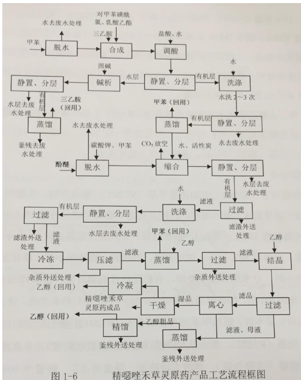
图 3.4.4-1 精恶唑禾草灵产品项目生产工艺流程图
