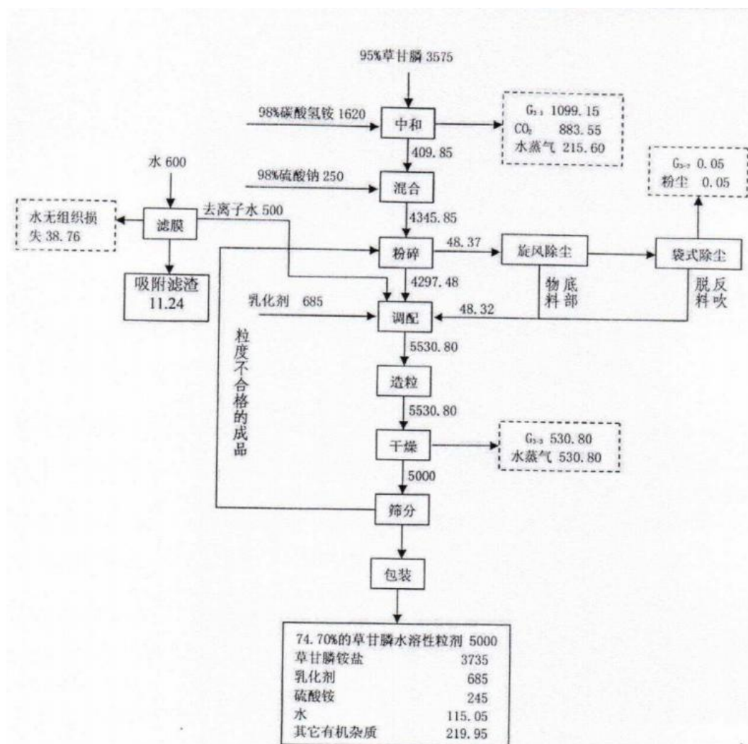
图 3.2-3 年产 5000 吨 74.7%草甘膦水溶性粒剂过程物料平衡图 单位：t/a
